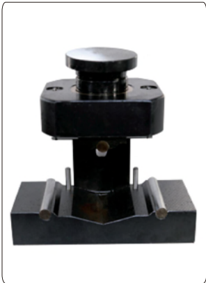
水泥胶砂抗折夹具(标配)
